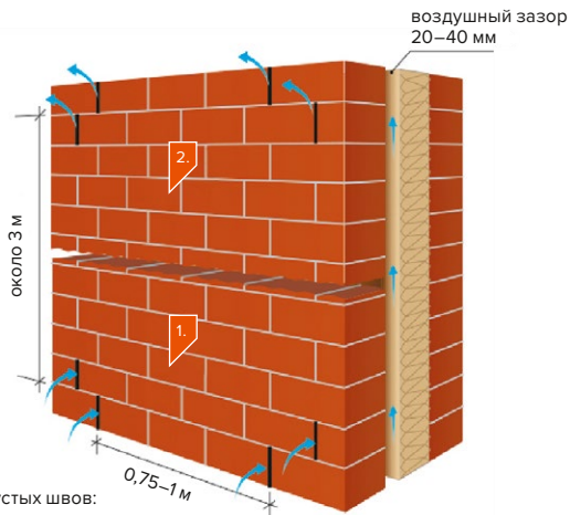
Рис. 2.5. Обеспечение притока и оттока воздуха при помощи продухов в конструкции слоистой кладки
