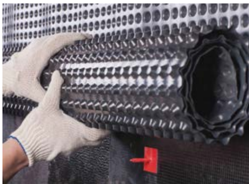
Защита гидро- изоляции
