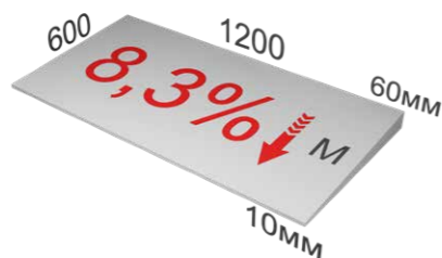
Плиты М с уклоном 8,3 %
