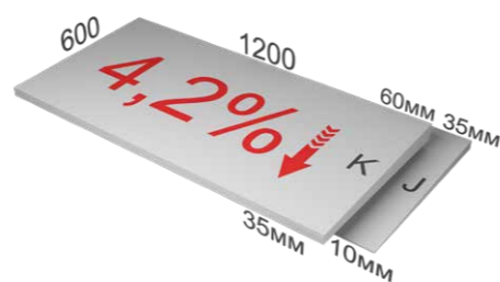
Плиты J и K с уклоном 4,2 %
