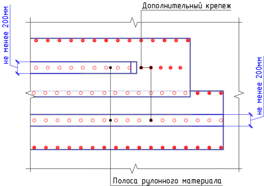
Рисунок 7.2 – Дополнительное крепление материала по его центральной оси
