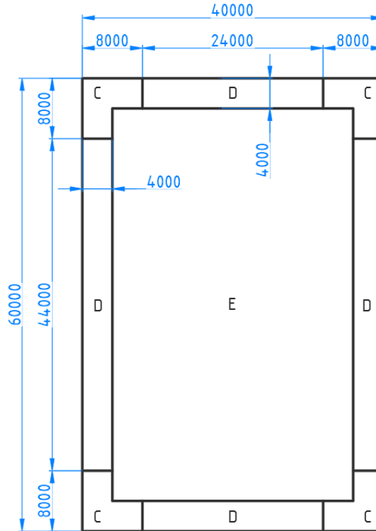
Рисунок Б.2 – План крыши здания
