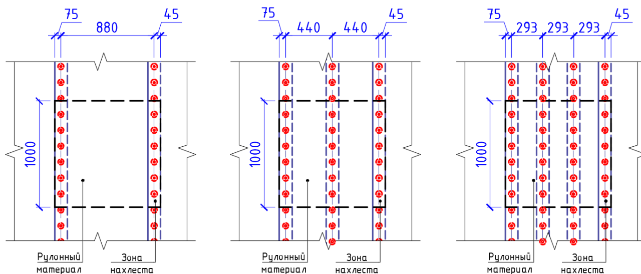
Рисунок Б.4– Нахлесты гидроизоляции
