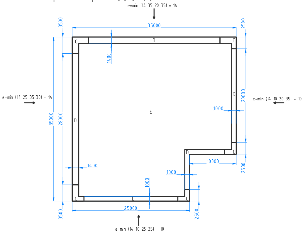
Рисунок Б.6 – План крыши здания
