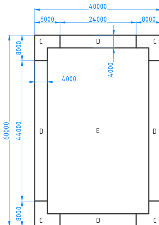
Рисунок Б.5 – План крыши здания
