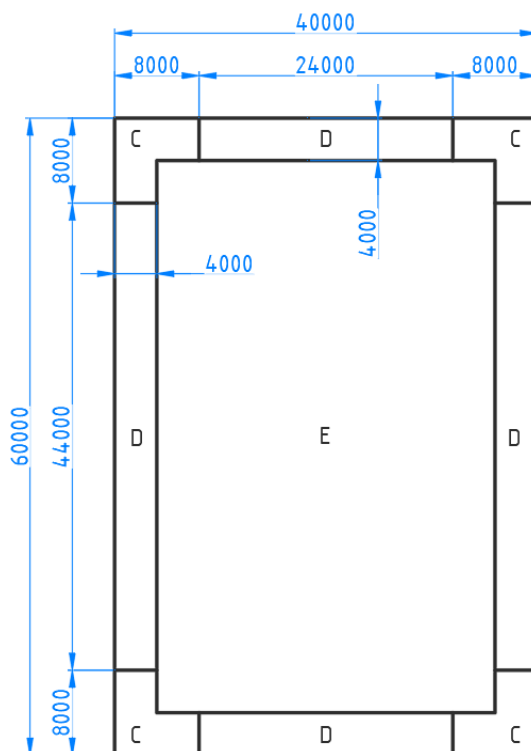
Рисунок Б.3– План крыши здания
