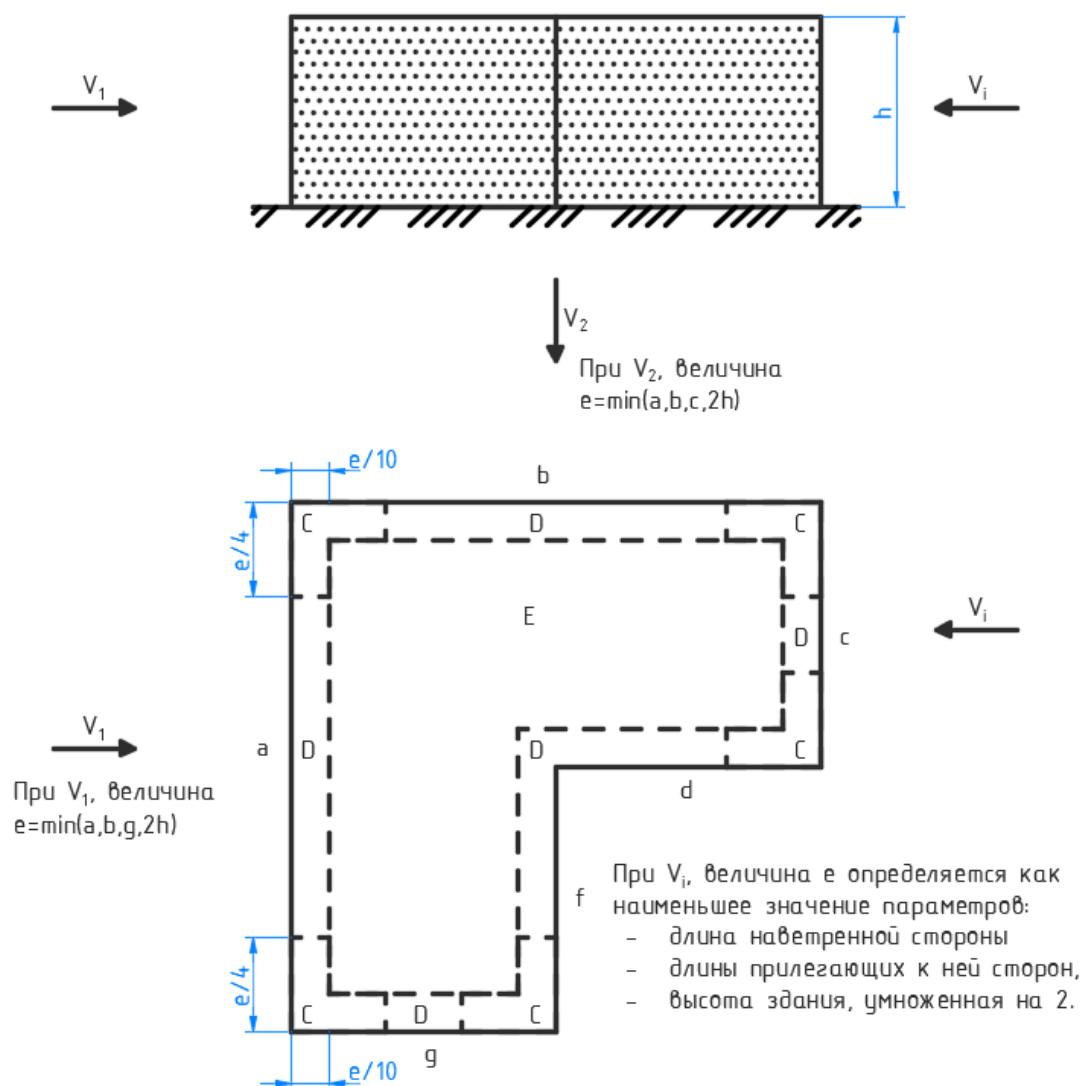
Рисунок 6.2 – Зоны плоских покрытий сложной геометрии
