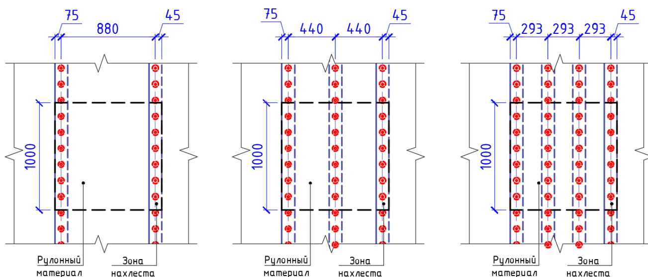
Рисунок Б.7 – Ширина шага между рядами крепления
