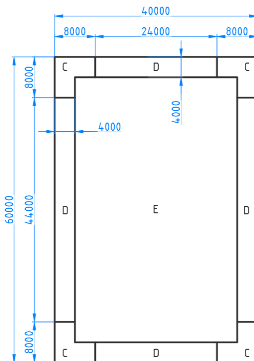
Рисунок Б.1 – План крыши здания
