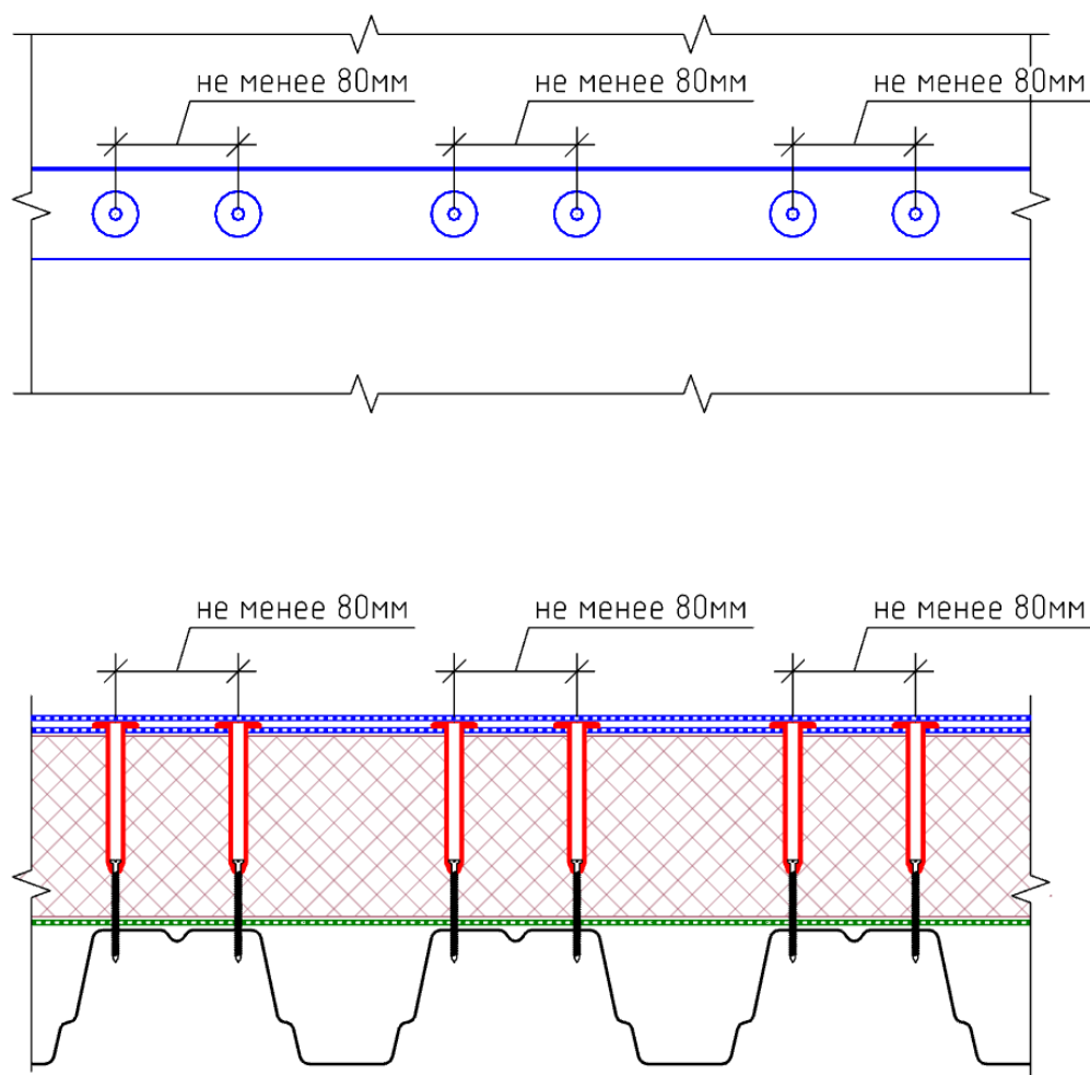
Рисунок 7.1 – Способ фиксации двойным креплением.
