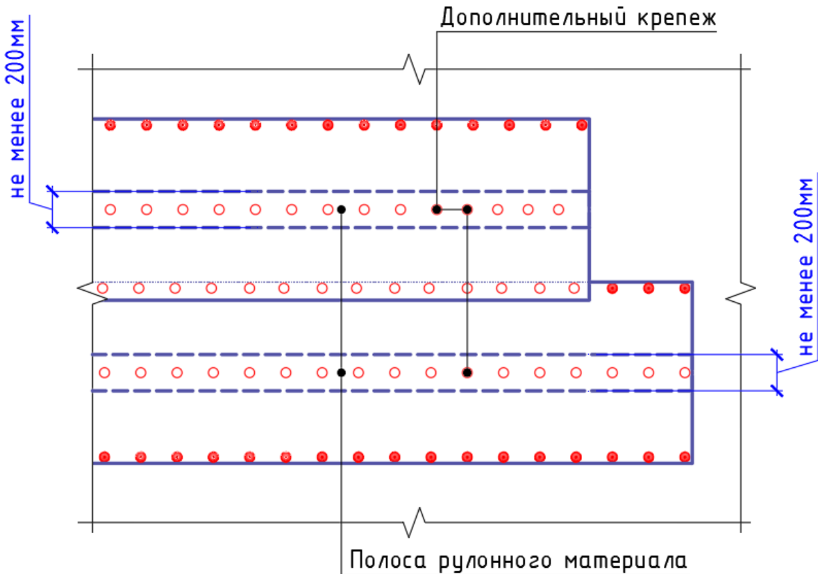
Рисунок 7.3 - Крепление слоя усиления для последующего наплавления водоизоляционного ковра
