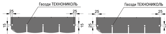
Рис. 5. Схема крепления фасадной плитки на 5 элементов крепежа
