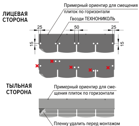
Рис. 4. Схема крепления фасадной плитки на 8 элементов крепежа
