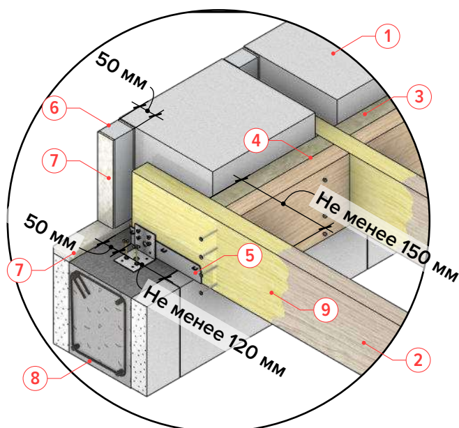
Узел 1. Опираие деревянных балок на внешнюю стену
