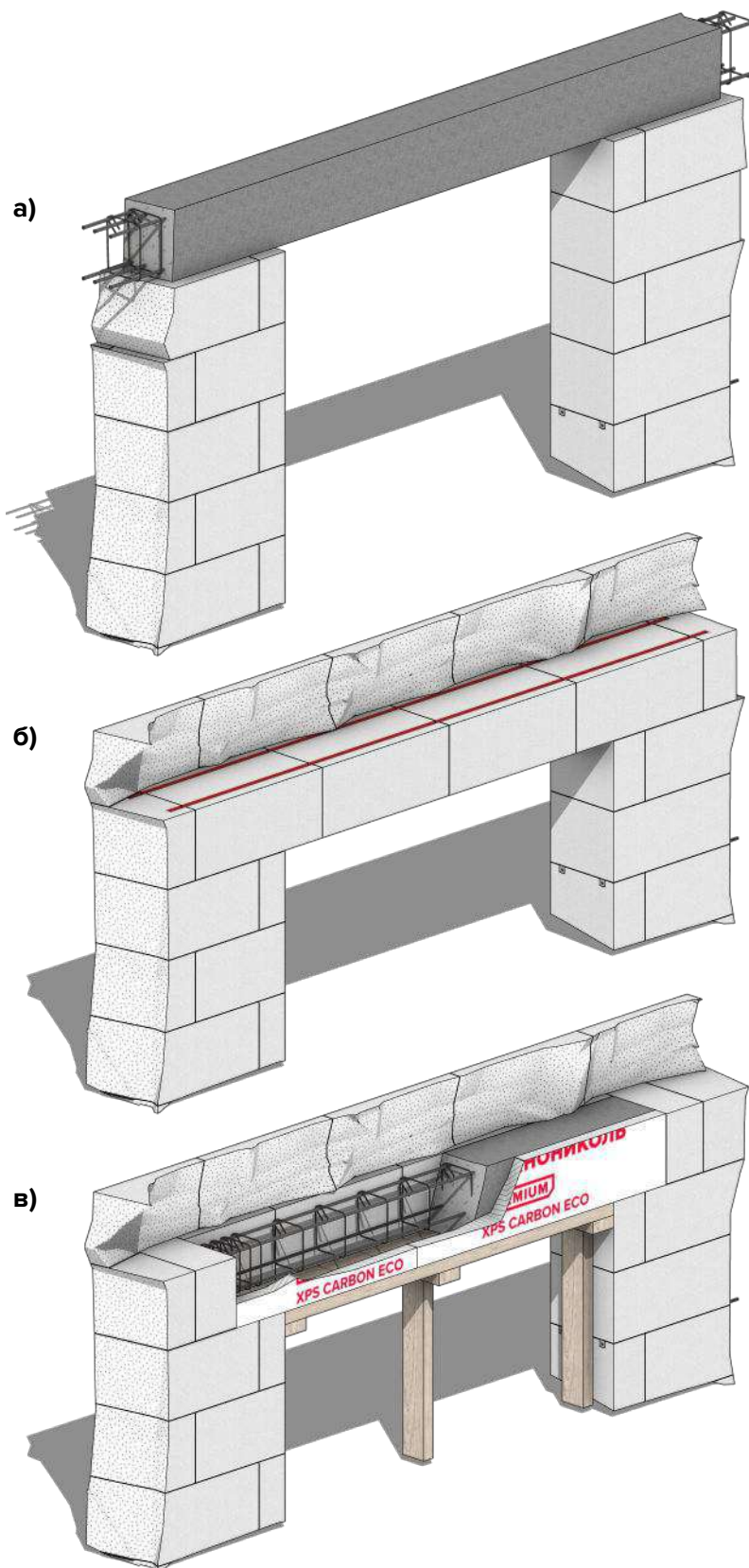
Рисунок 16. Варианты перемычек над проемом
