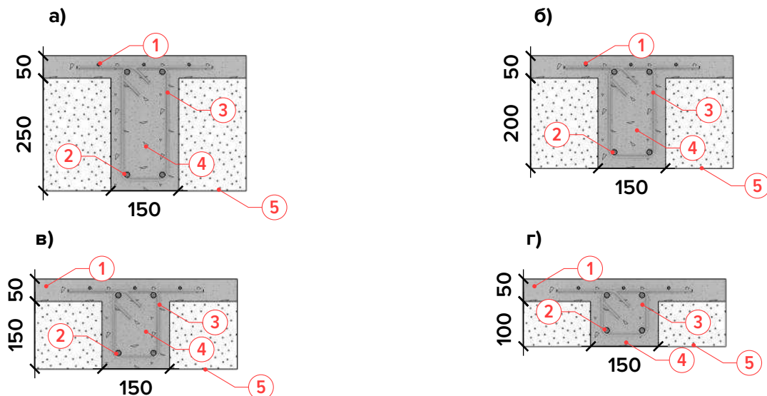
Рисунок 31. Типовое сечение ребер сборно-монолитного перекрытия
