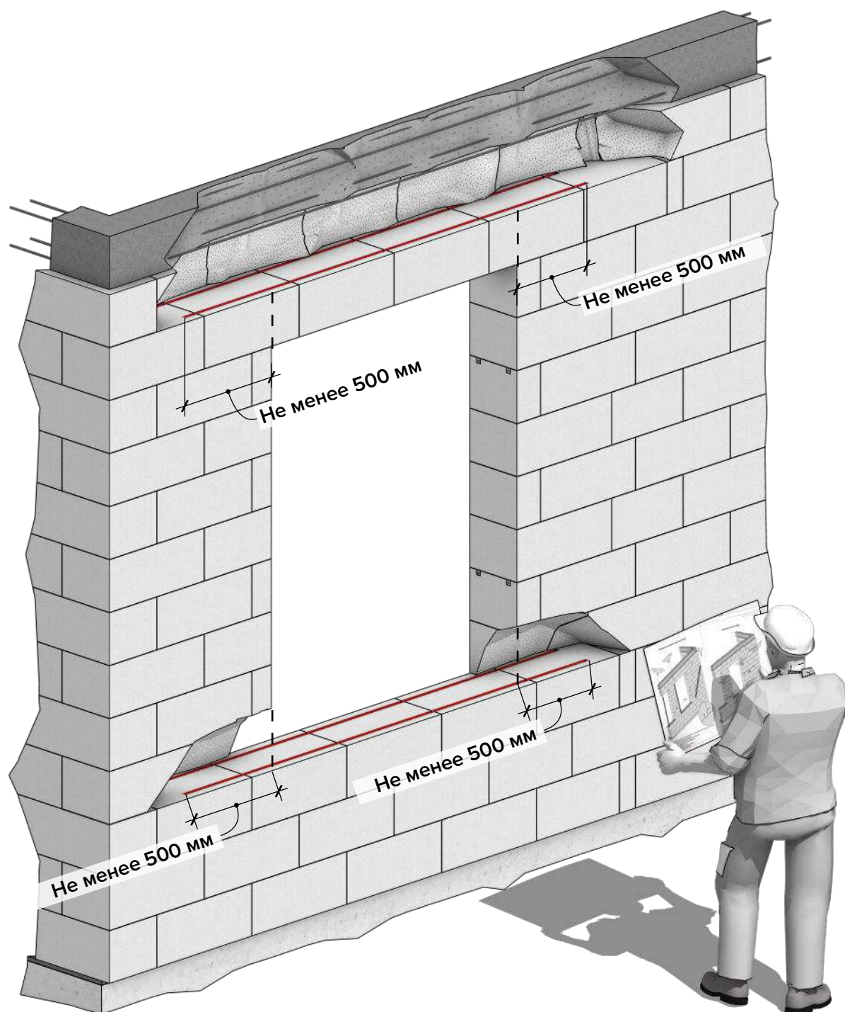
Рисунок 13. Армирование проемов
